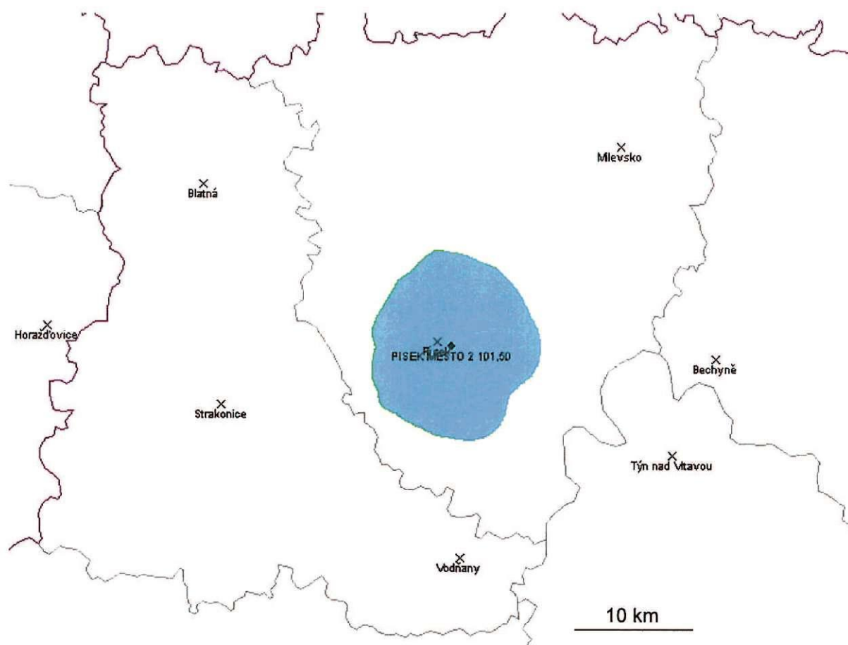
Diagram využití rádiového kmitočtu PISEK MESTO 2 101,5 MHz podle § 112 odst. 4 zákona 127/2005 o elektronických komunikacích.
