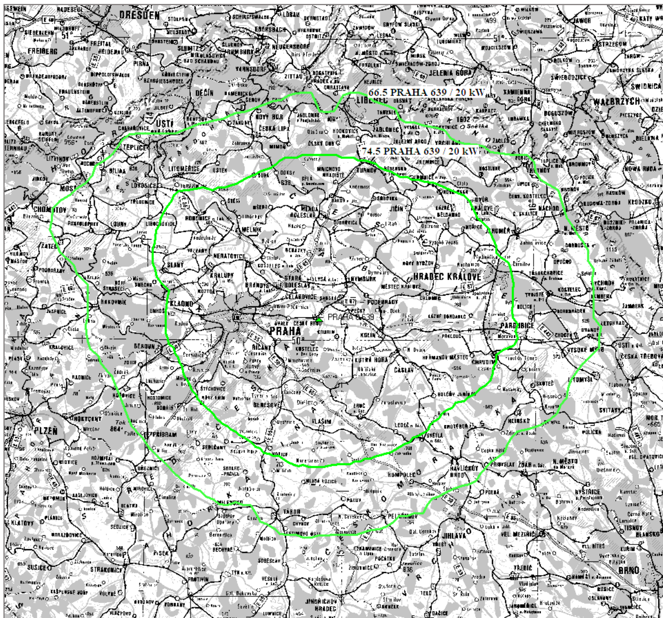
Diagram využití kmitočtu PRAHA 639 kHz / 20 kW daný nominální použitelnou intenzitou pole přízemní složky elektromagnetické vlny E_u = 66,5 \text{ dB}_\mu (den) a 74,5 \text{ dB}_\mu (noc – venkov).
