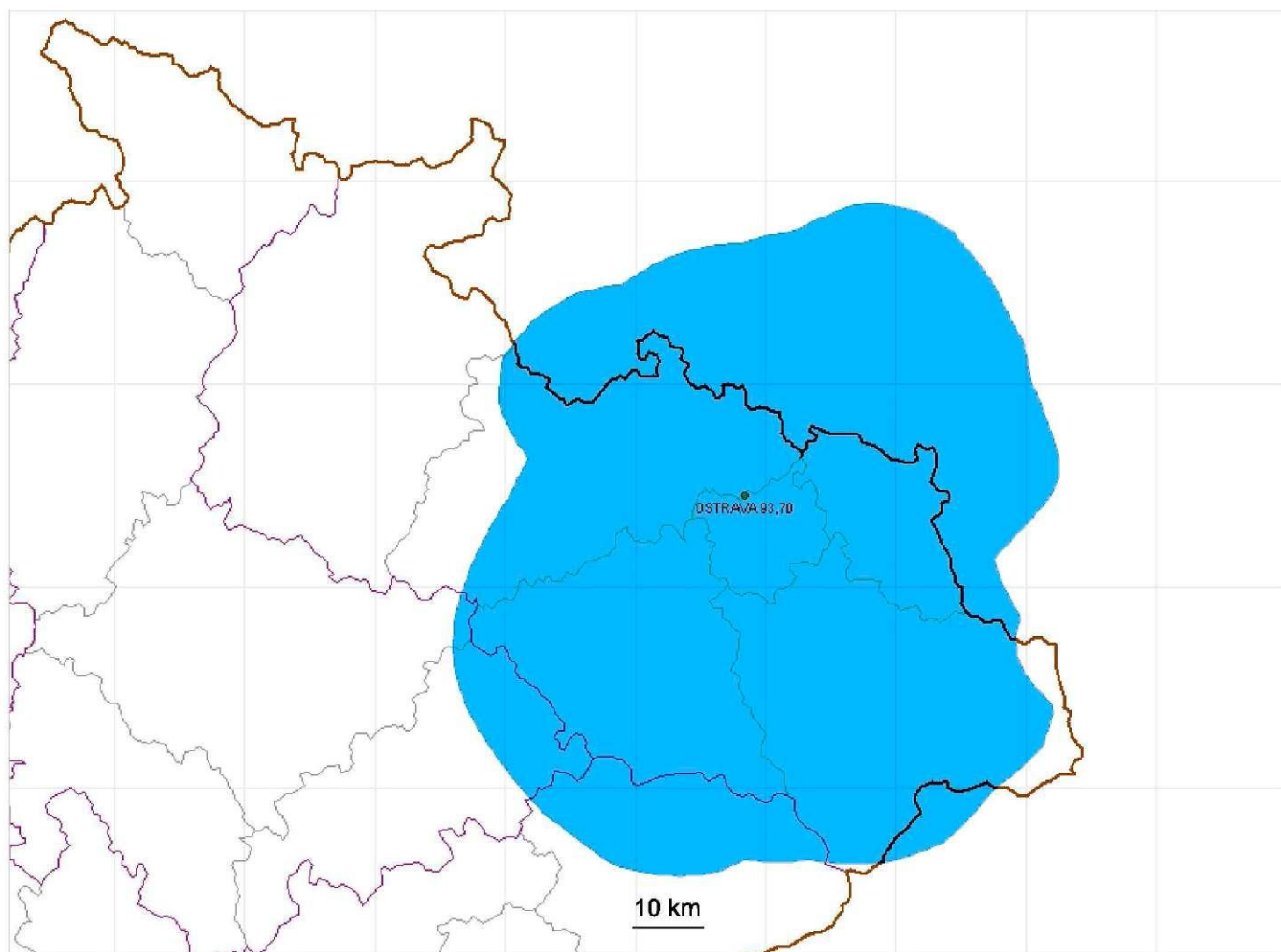
Diagram využití rádiového kmitočtu OSTRAVA 93,7 MHz stanovený výpočtem podle vyhlášky č. 22 / 2011 Sb. o způsobu stanovení pokrytí signálem zemského rozhlasového vysílání ve vybraných kmitočtových pásmech – modrá barva.
