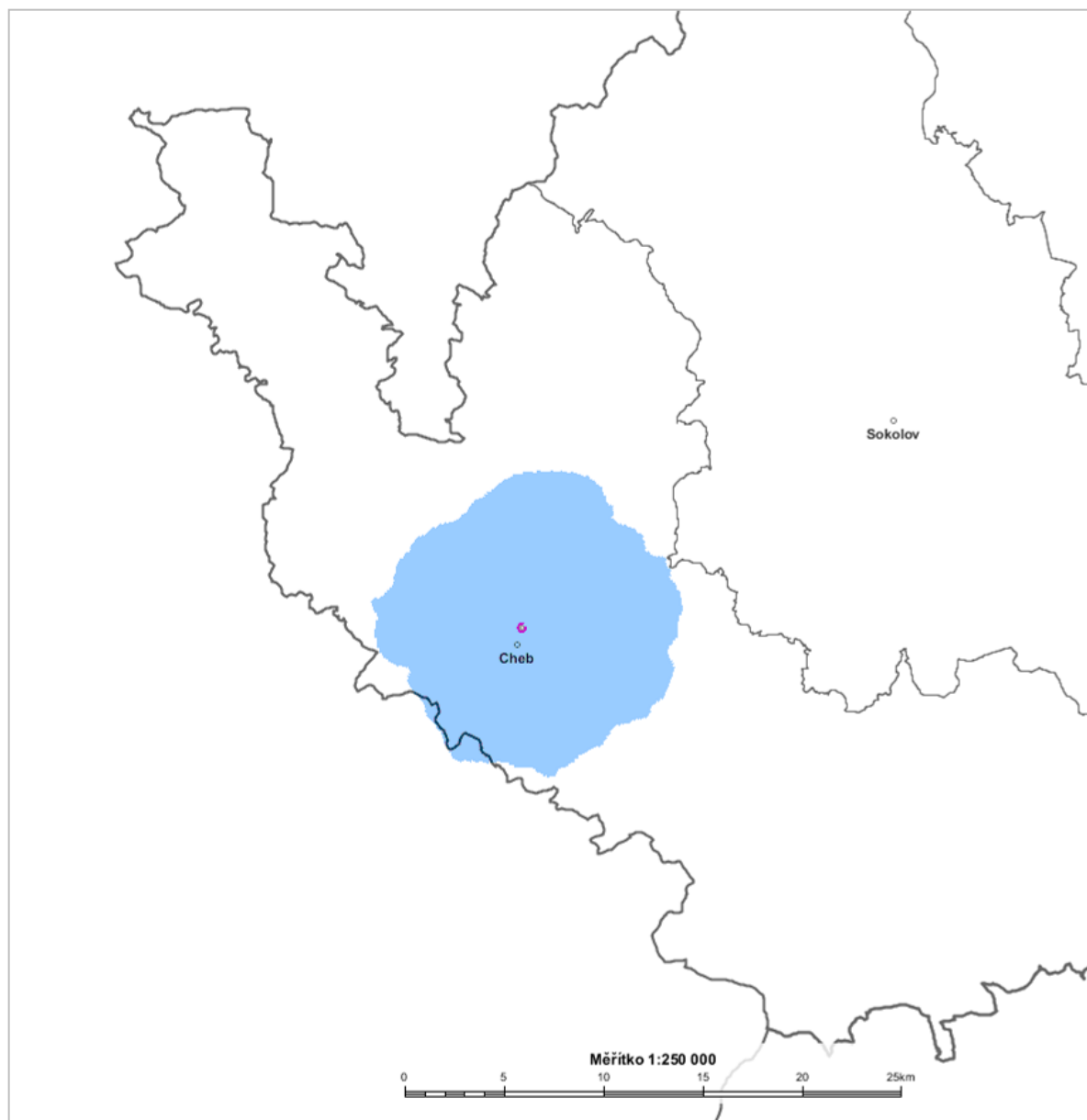
Diagram využití rádiových kmitočtů určených pro analogové vysílání v pásmu VKV pro vysílač CHEB 1 91,8 MHz stanovený výpočtem podle vyhlášky č. 22/2011 Sb. (modrá barva).
