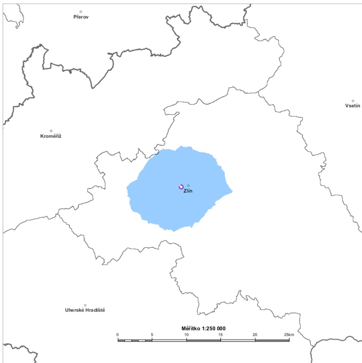
Diagram využití rádiových kmitočetů určených pro analogové vysílání v pásmu VKV pro vysílač ZLIN 5 88,6 MHz stanovený výpočtem podle vyhlášky č. 22/2011 Sb. (modrá barva).
