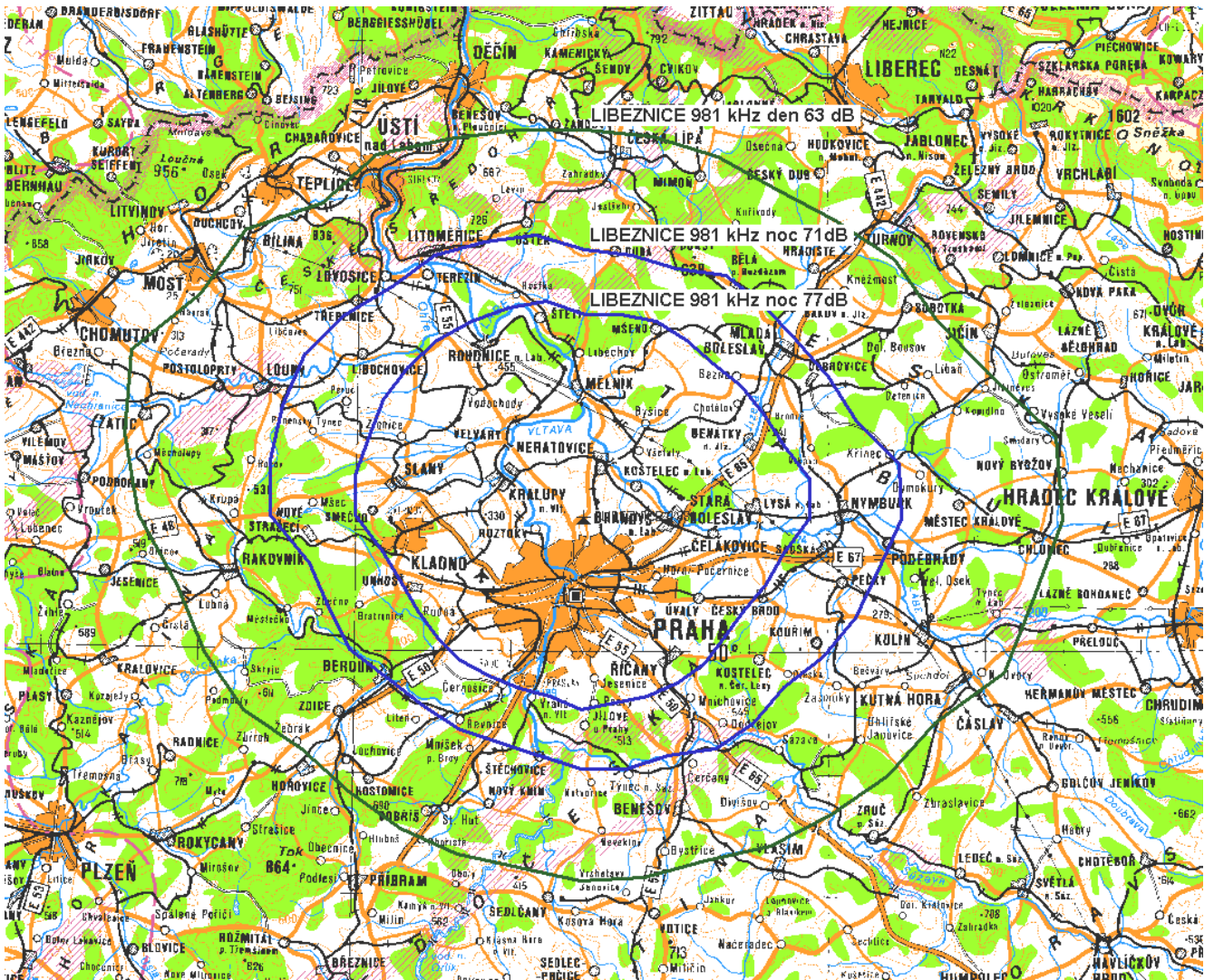
Diagram využití kmitočtu LIBEZNICE 981 kHz / 40 dBW daný nominální použitelnou intenzitou pole přízemní složky elektromagnetické vlny E_u .
