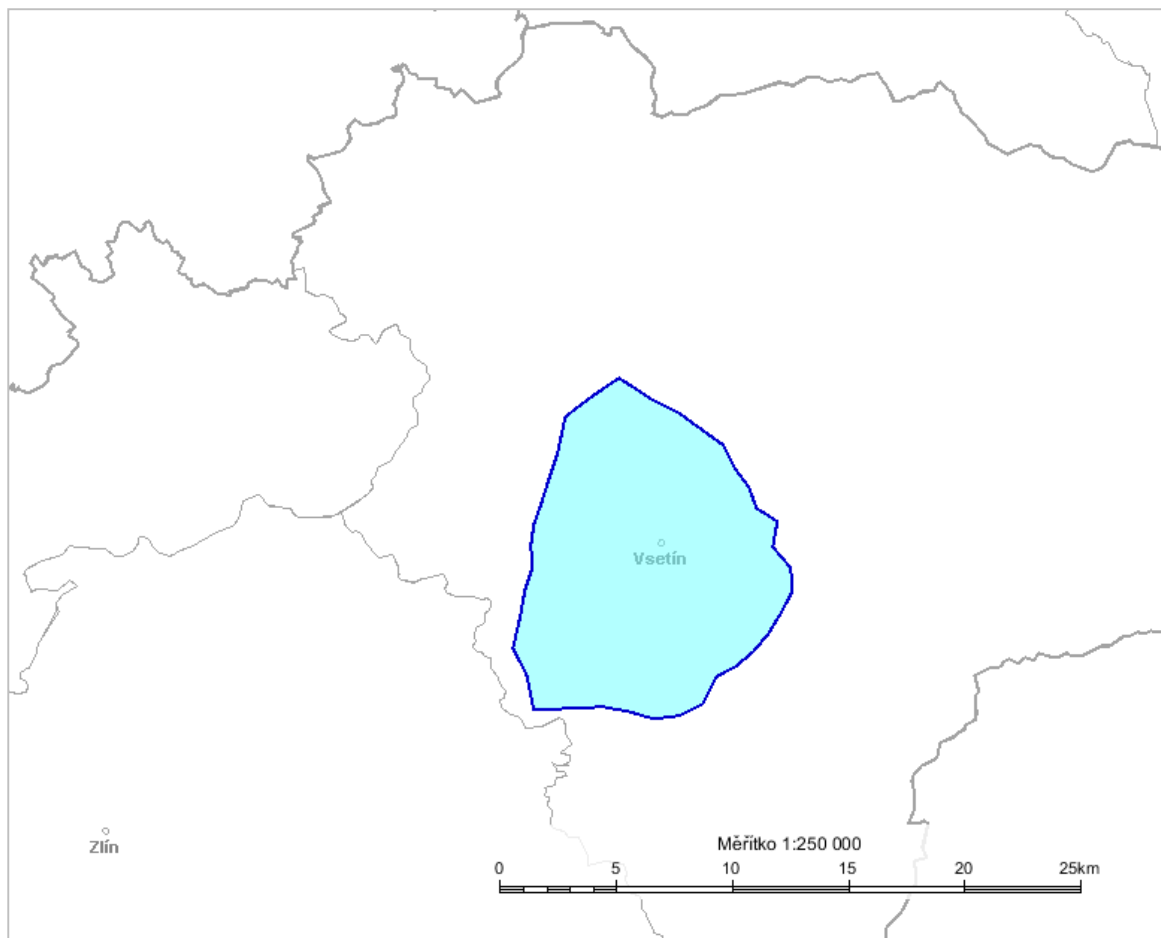
Diagram využití rádiového kmitočtu VSETIN 93,5 MHz stanovený výpočtem podle vyhlášky č. 22/2011 Sb. o způsobu stanovení pokrytí zemského rozhlasového vysílání ve vybraných kmitočtových pásmech – modrá barva.
