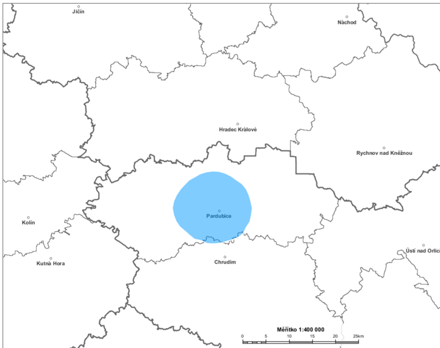
Diagram využití rádiových kmitočtů určených pro analogové vysílání v pásmu VKV pro vysílač PARDUBICE POLABINY 94,5 MHz stanovený výpočtem podle vyhlášky č. 22/2011 Sb. (modrá barva).
