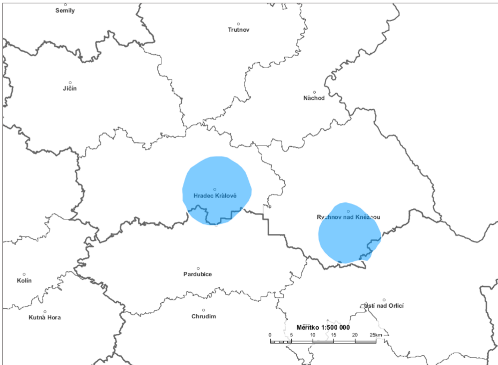
Diagram využití rádiových kmitočtů určených pro analogové vysílání v pásmu VKV pro vysílače HRADEC KRALOVE 3 105,1 MHz a VAMBERK 2 92,4 MHz stanovený výpočtem podle vyhlášky č. 22/2011 Sb. (modrá barva).
